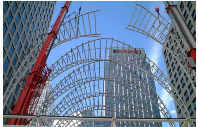
Montage der Binderkonstruktionen
